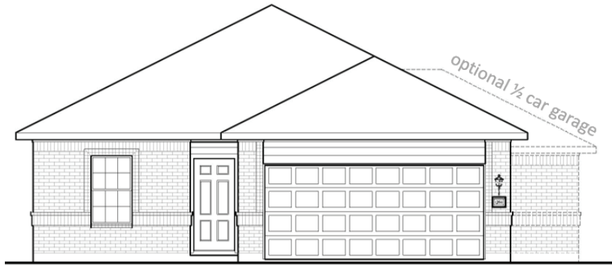
ELEVATION A
