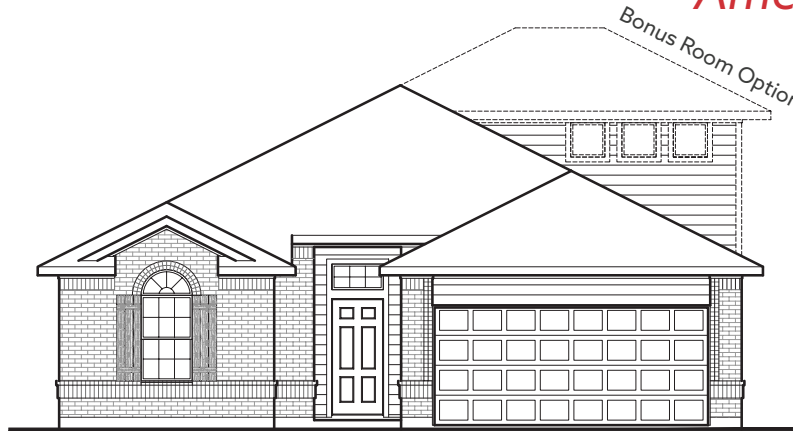
ELEVATION A
